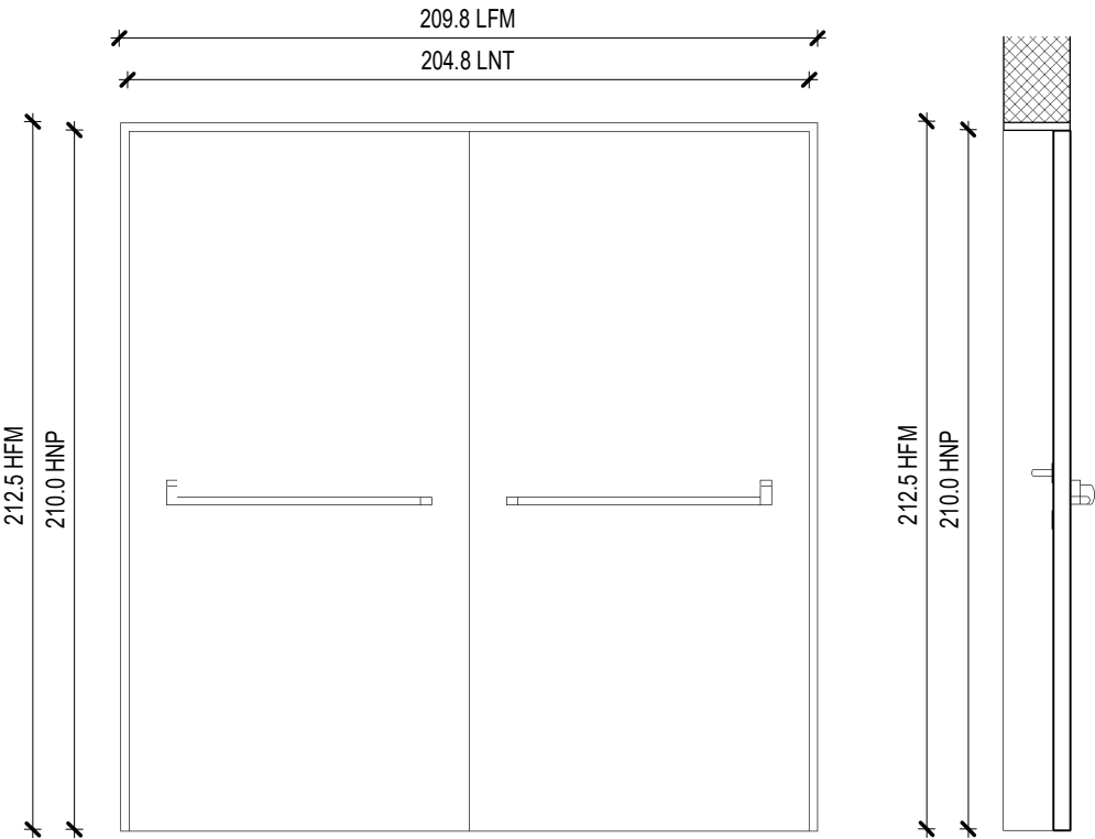
Prospetto
