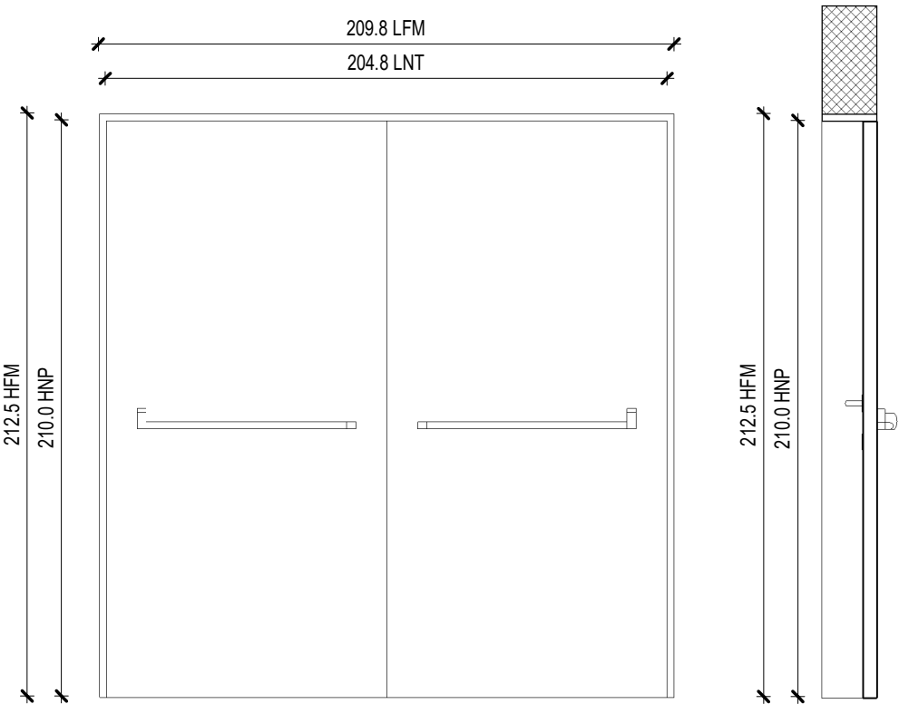
Prospetto
