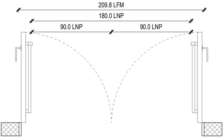
Pianta
