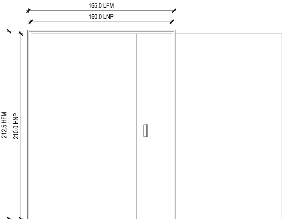
Prospetto
