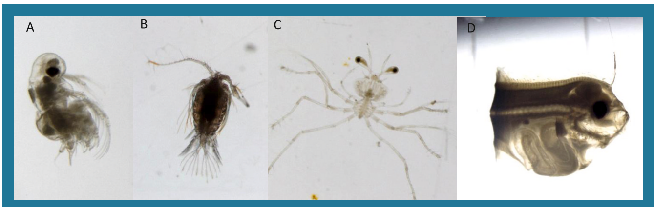
Figura 3. Immagini acquisite allo stereomicroscopio di alcune specie di mesozooplankton rinvenute nel 2024. A) Podon leuckartii (gruppo Cladoceri); B) Pontellina plumata (gruppo Copepodi); C) larva phyllosoma; D) Larva di pesce cfr. Arnoglossus thori .
