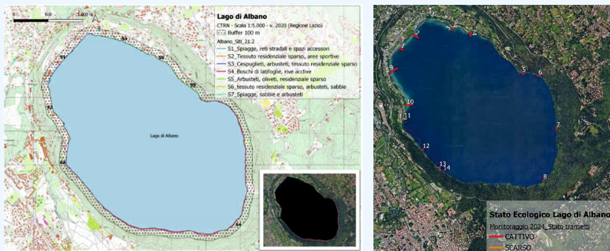
Figura 4. Lago di Albano: a sinistra mappa d'individuazione dei Siti con ausilio di CTR 1:5000 (fonte Regione Lazio); a destra mappa dei transetti campionati nell'anno 2024 colorati in base al corrispondente giudizio di qualità di Stato Ecologico.
