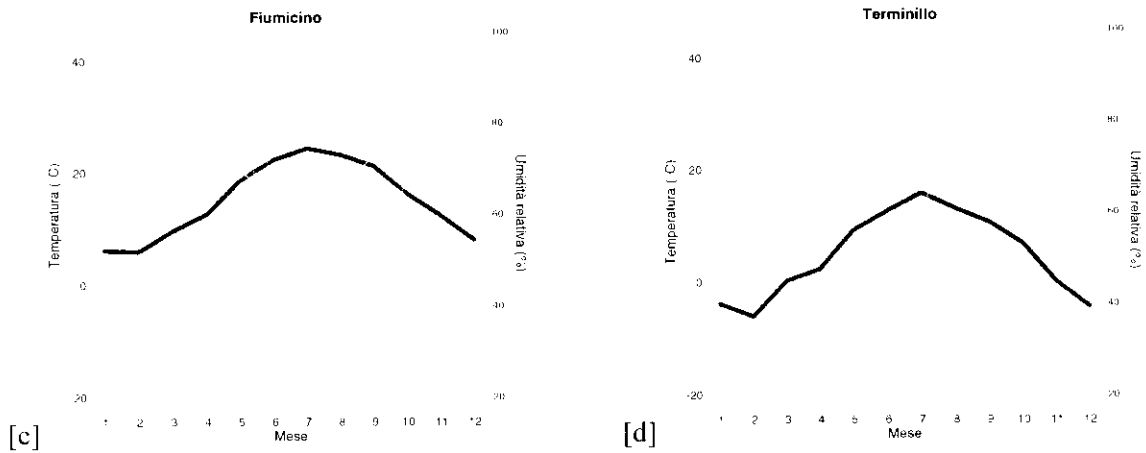
Figura 2.48 - Valori Medi, minimi e massimi mensili della temperatura e valori medi dell'umidità relativa rilevate nel 2005 dalle stazioni dell'Aeronautica.
