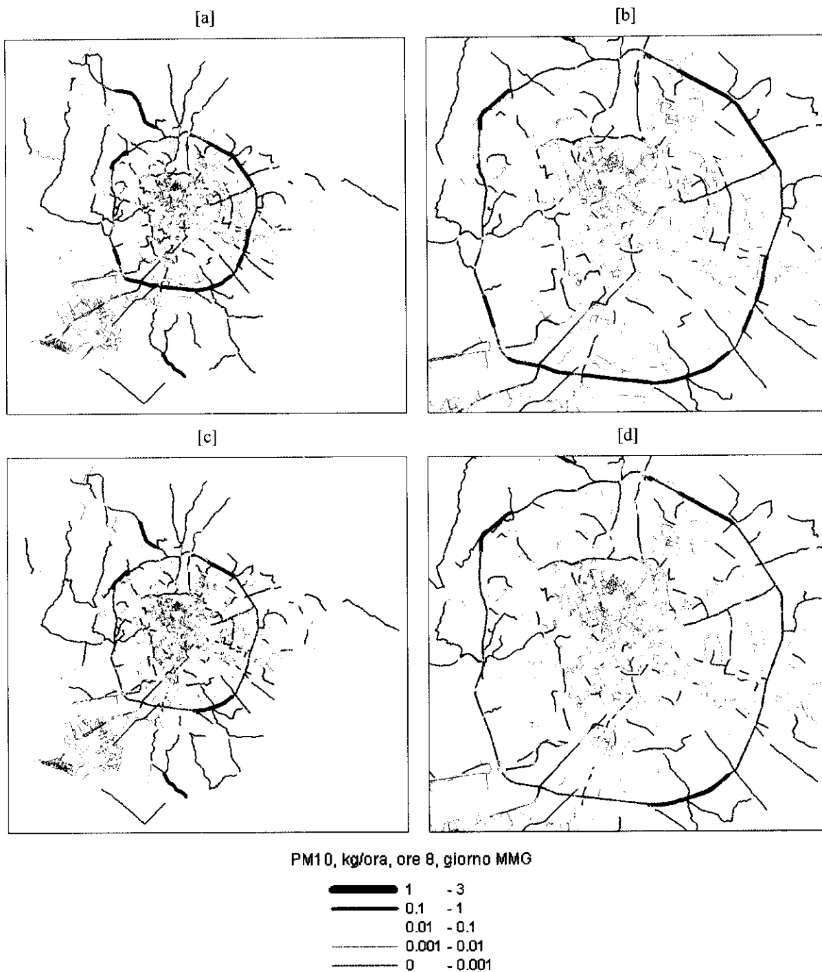
Figure 6.25, a, b, c, d: mappa tematica delle emissioni di PM10 nell'ora di punta della mattina (8), nel giorno tipo MMG, nello scenario attuale (sopra) e futuro (sotto). L'unità di misura è il chilogrammo. Sulla sinistra la rete completa, sulla destra l'ingrandimento della zona interna al GRA.
