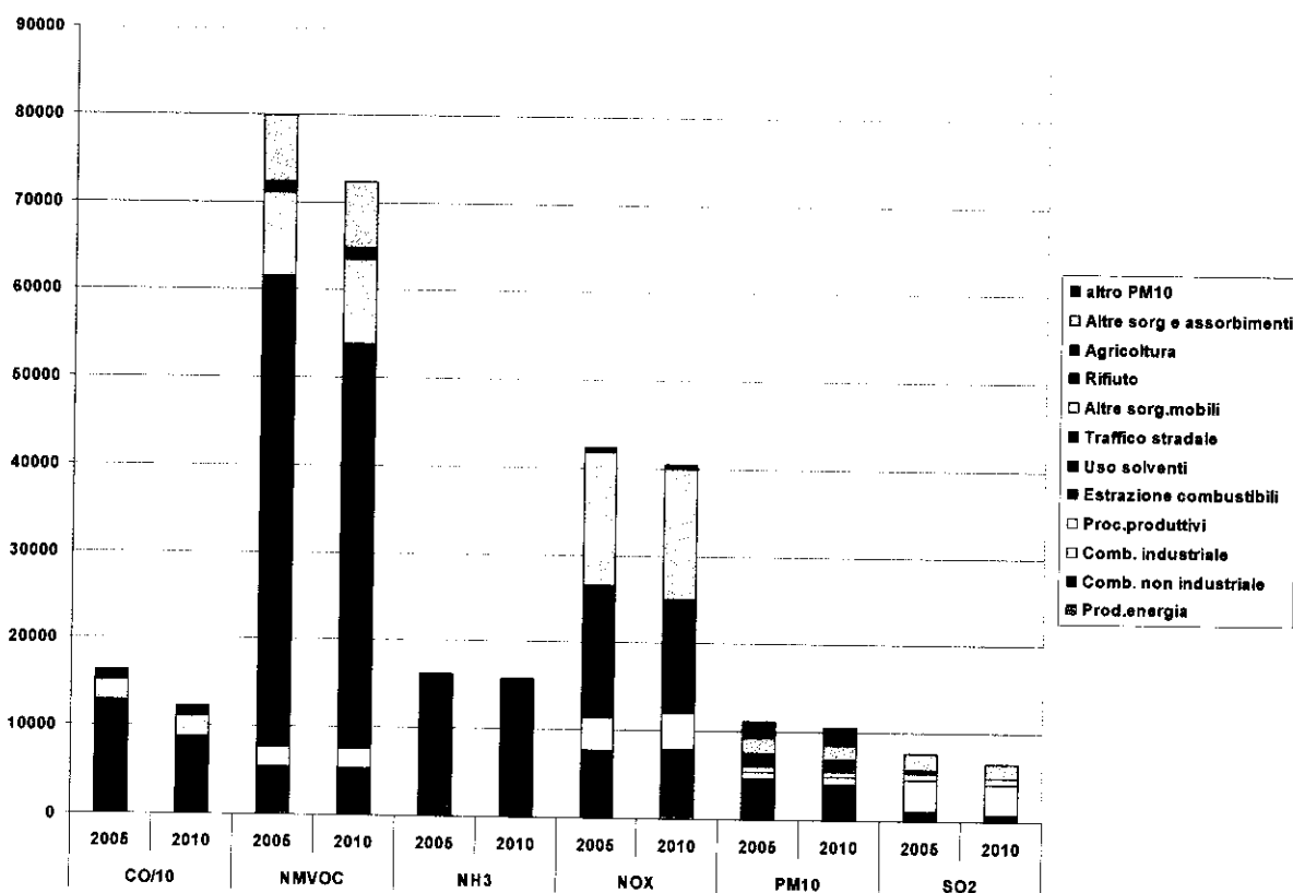
Figura 6.6 – Trend delle emissioni regionali diffuse (t/anno) dal 2005 al 2010.
