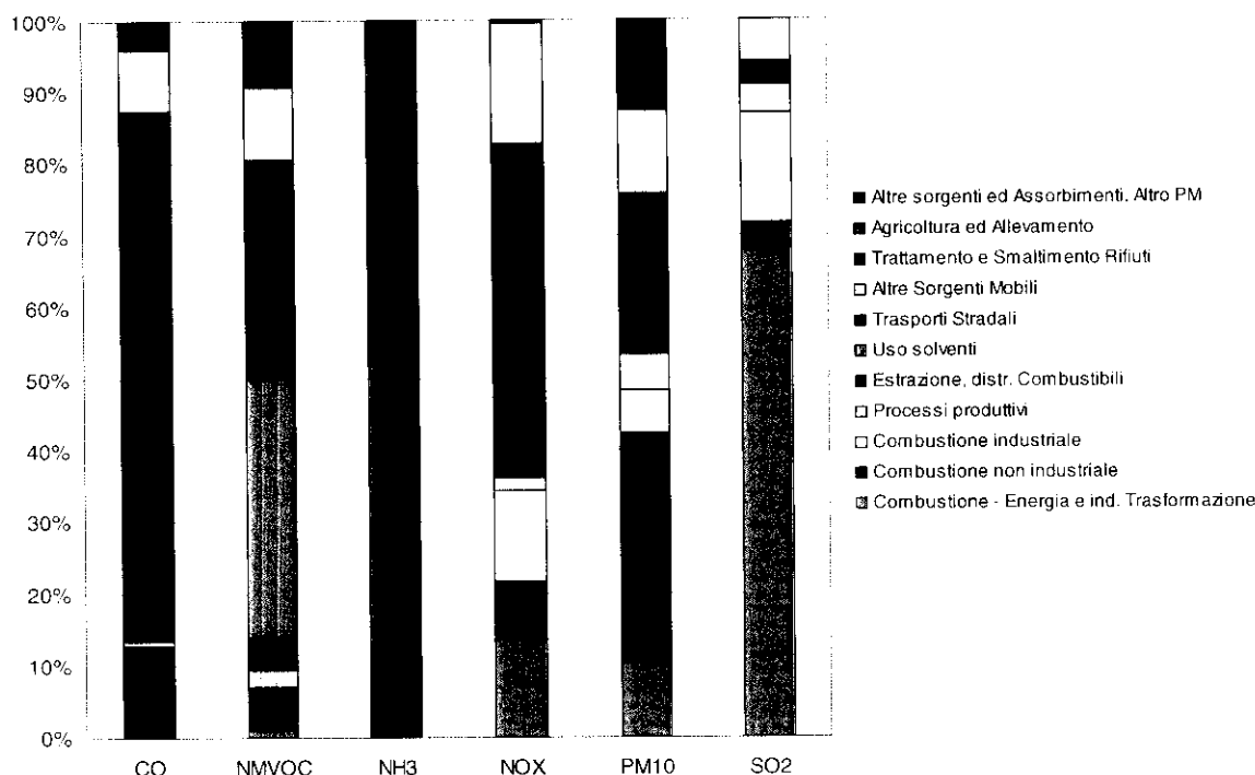
Figura 2.25 – Emissioni percentuali totali sul territorio regionale.
