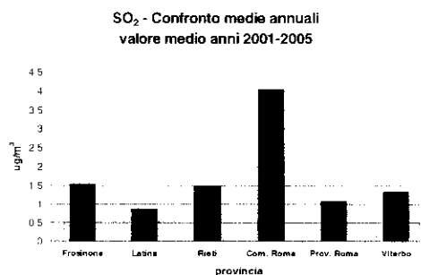
Figura 2.59 - Valore medio della concentrazione annuale di biossido di zolfo per provincia.
