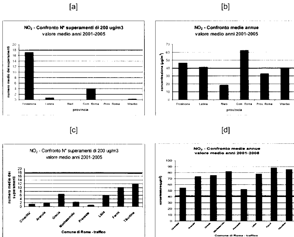
Valore medio del numero di superamenti (a) e della concentrazione annuale (b) di NO 2 . La linea rossa rappresenta il limite di legge dei 18 superamenti annuali (a) e di 40 µg/m 3 per la media annua (b).
