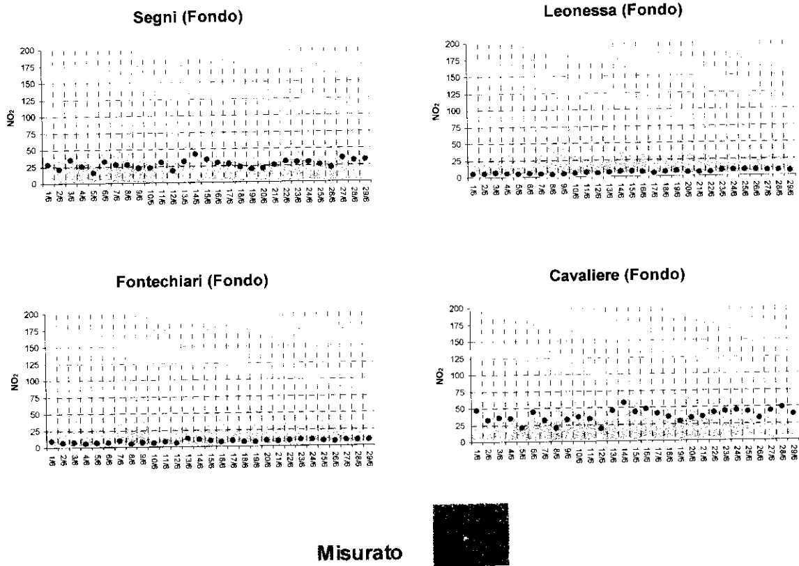
Figura 3.35 – Concentrazioni medie giornaliere osservate e calcolate di NO 2 [µg m -3 ] relativamente al mese di giugno 2005 in stazioni di fondo (dominio regionale).
