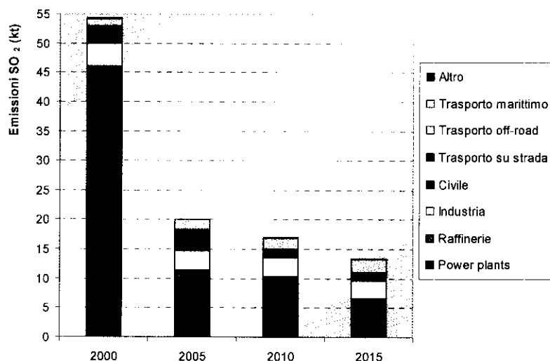
Figura 6.1 – Emissioni SO 2 - scenario CLE - LAZIO.
