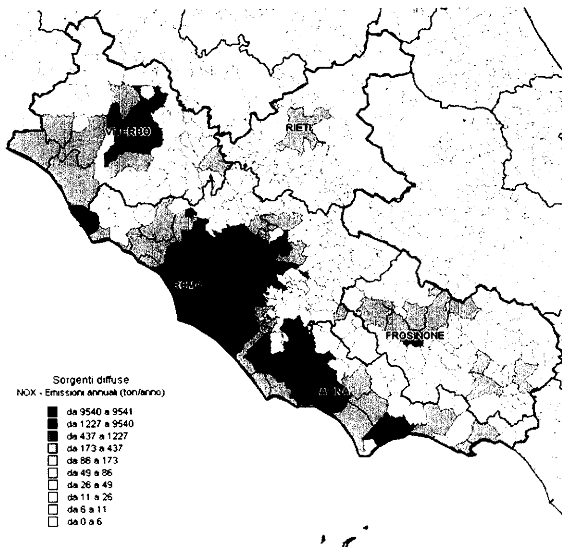
Figura 2.3 – Emissioni diffuse di \text{NO}_x della regione Lazio (tenuto conto dell'assenza della parte di traffico urbano del comune di Roma).
