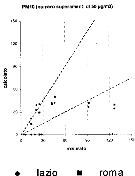
Figura 3.48 – Standard di Qualità dell'aria: Numero di superamenti del valore limite per le concentrazioni medie giornaliere di PM10 (Valore limite per la protezione della salute: 50 µg m-3 da non superare più di 35 volte per anno civile
