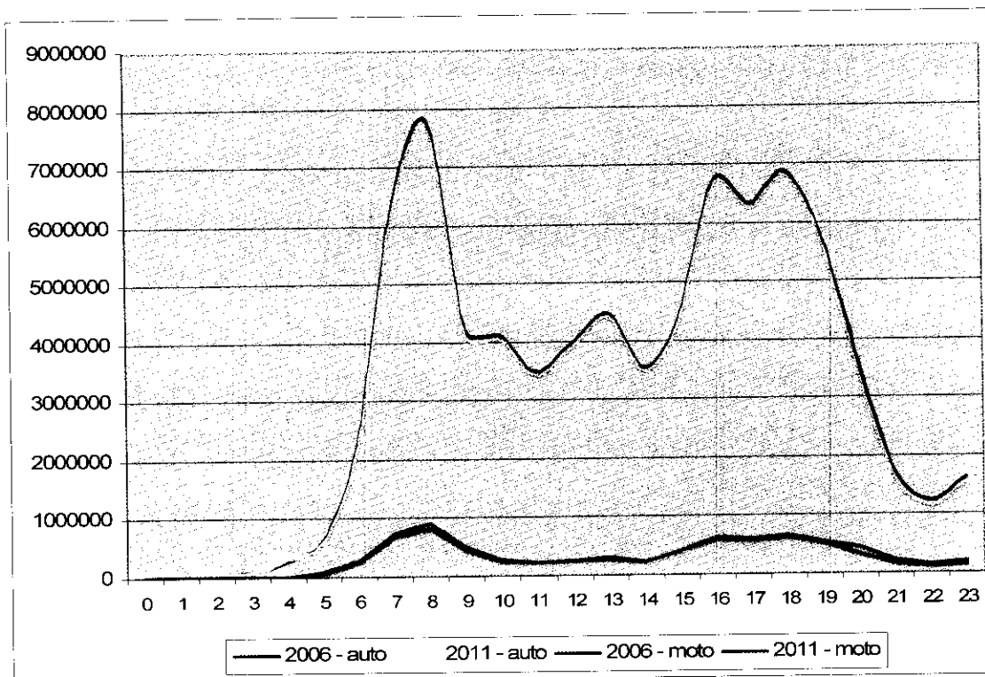
Figura 6.16 : curva oraria del traffico sull'intera rete, nel giorno tipo MMG, per auto e moto, nei due scenari
