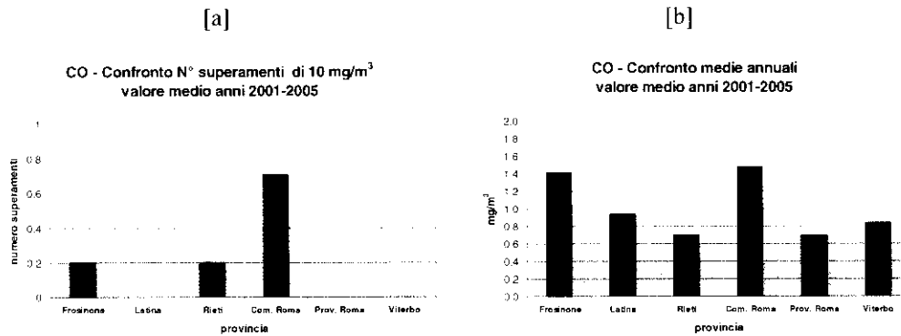
Figura 2.56 - Valore medio del numero di superamenti e della media annuale della concentrazione del monossido di carbonio per provincia.
