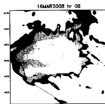
Figura 1.6 Mappe di previsione a breve termine delle concentrazioni di inquinanti
