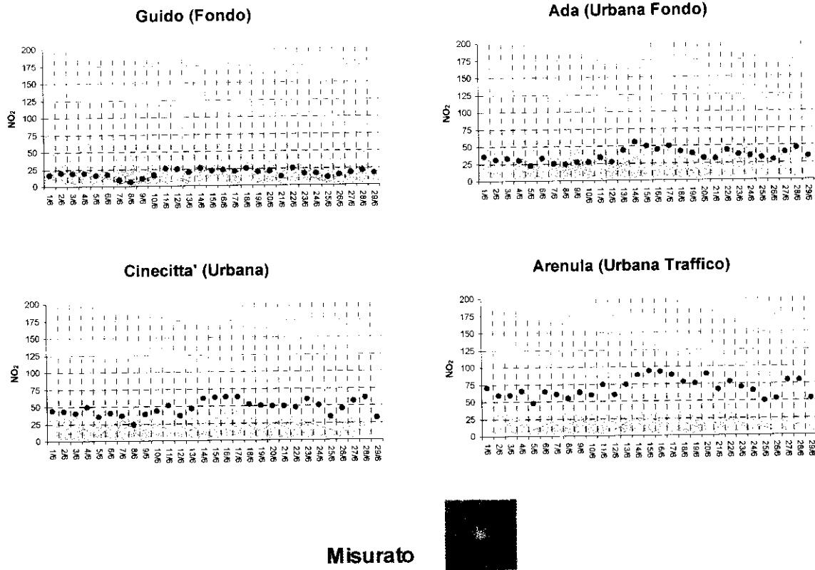
Figura 3.33 – Concentrazioni medie giornaliere osservate e calcolate di NO 2 [µg m -3 ] relativamente al mese di giugno 2005 (dominio locale).
