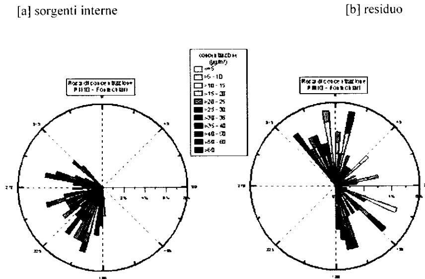
Figura 2.28 – Rose di concentrazione del PM_{10} misurata a Fontechiari in funzione alla direzione di provenienza del vento rilevata a 1000 m.
