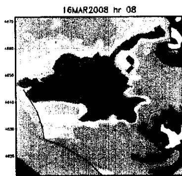
Figura 1.6 Mappe di previsione a breve termine delle concentrazioni di inquinanti
