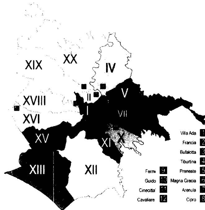
Figura 2.53 - Localizzazione delle stazioni di misura della rete automatica della qualità dell'aria nel comune di Roma.
