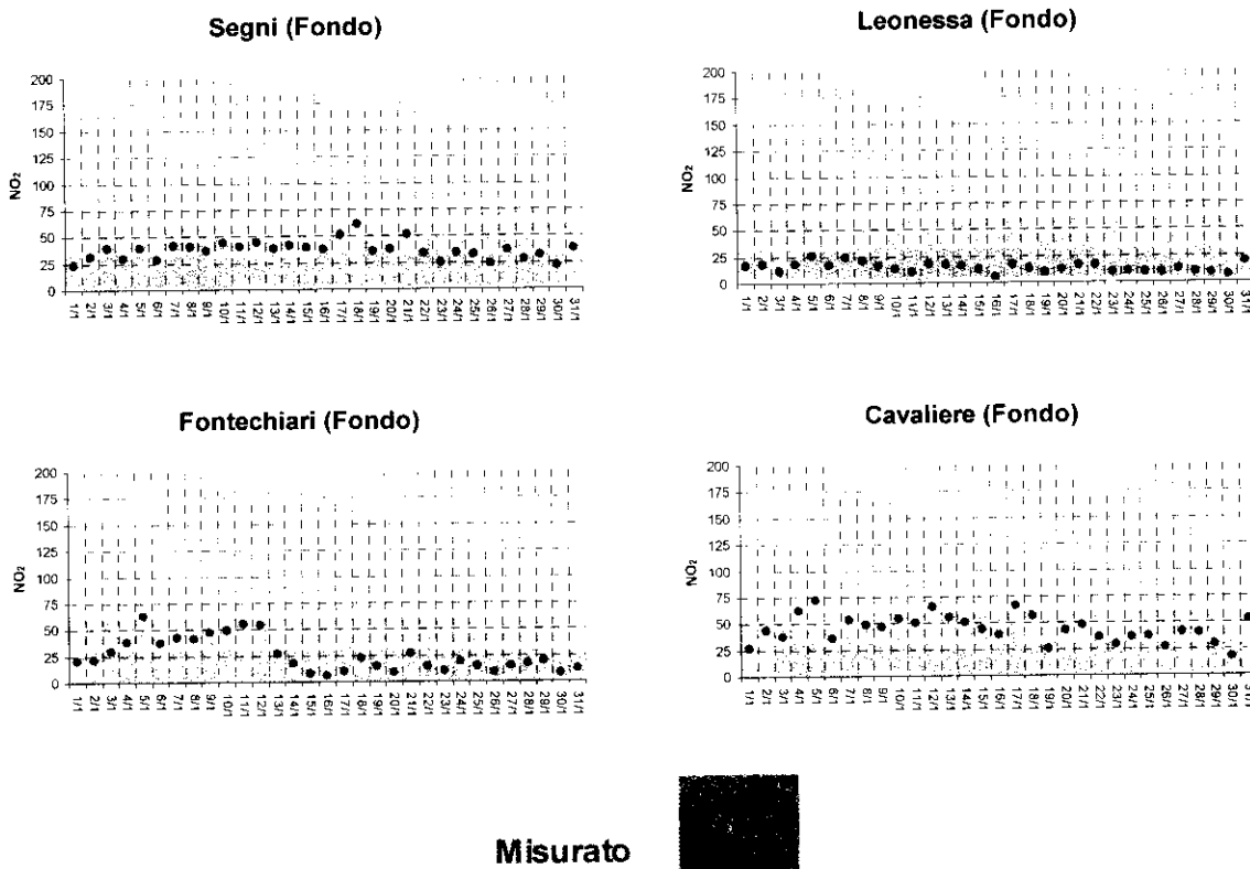
Figura 3.34 – Concentrazioni medie giornaliere osservate e calcolate di NO 2 [µg m -3 ] relativamente al mese di gennaio 2005 in stazioni di fondo (dominio regionale).
