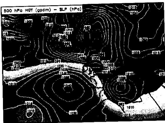
Figura 3.13 - 19 gennaio 2005: 13:00, geopotenziale a 500 HPa e pressione a livello del mare (sinistra) e immagine METEOSAT (destra).
