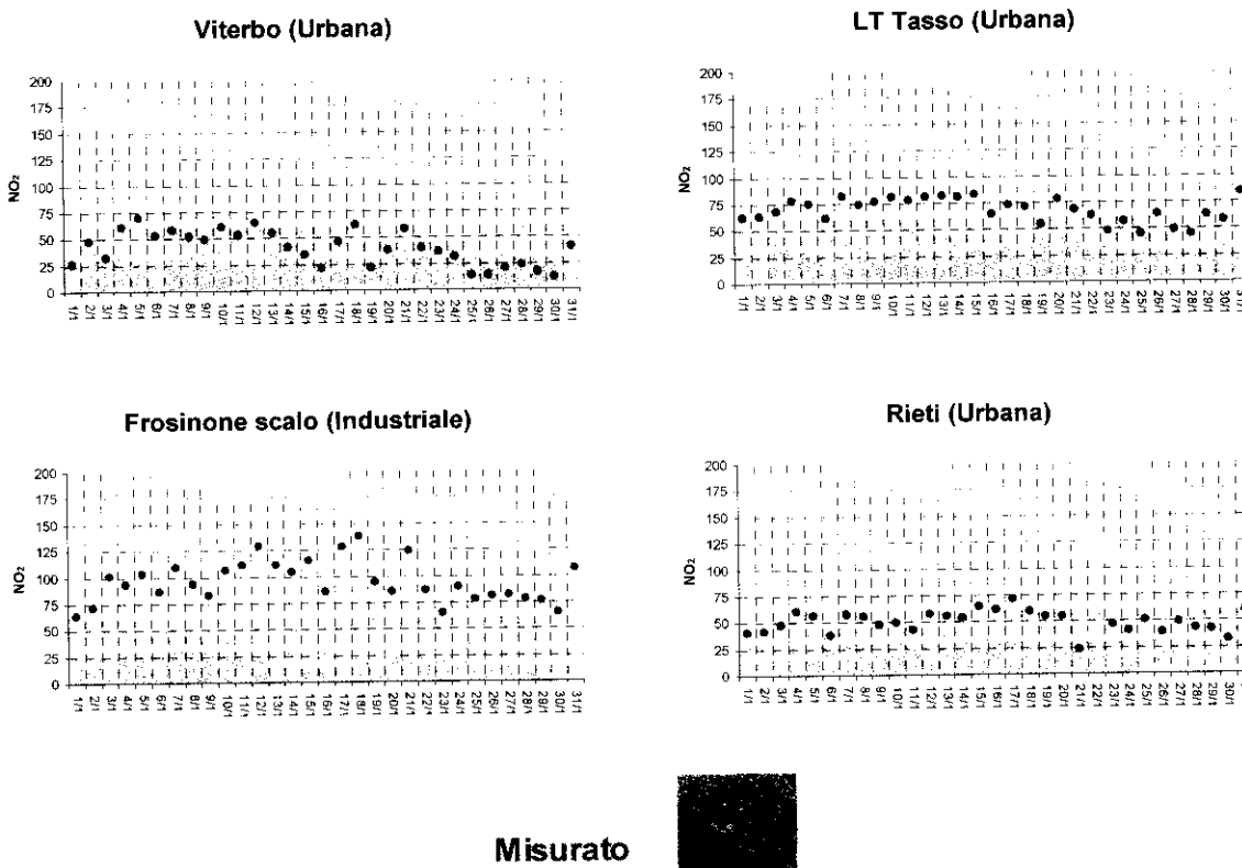
Figura 3.36 – Concentrazioni medie giornaliere osservate e calcolate di NO 2 [µg m -3 ] relativamente al mese di gennaio 2005 (dominio regionale).
