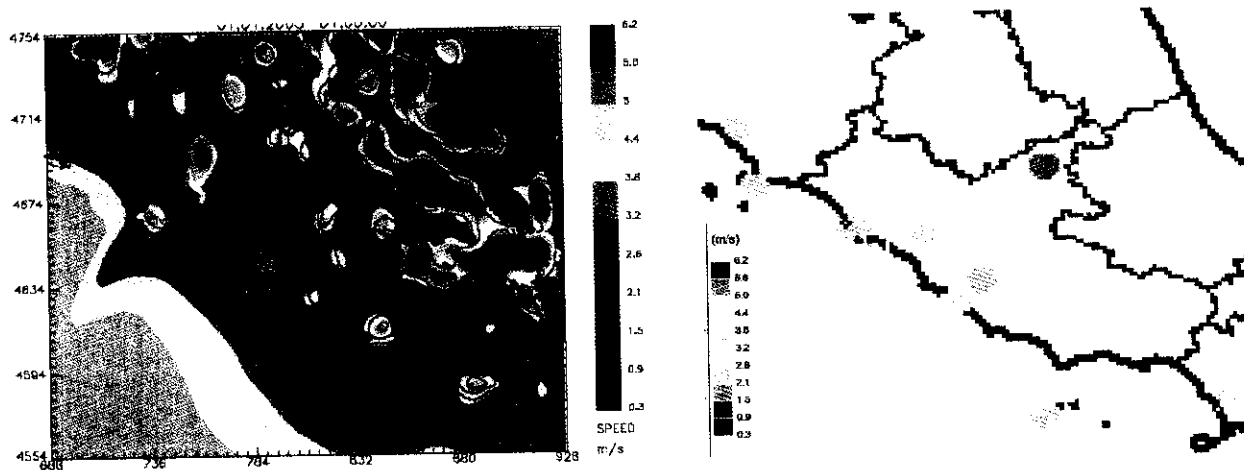
Figura 3.23 - Confronto tra i campi di vento al suolo (sinistra) e i dati SCIA di vento medio in prossimità del suolo (destra) relativi all'anno 2005.
