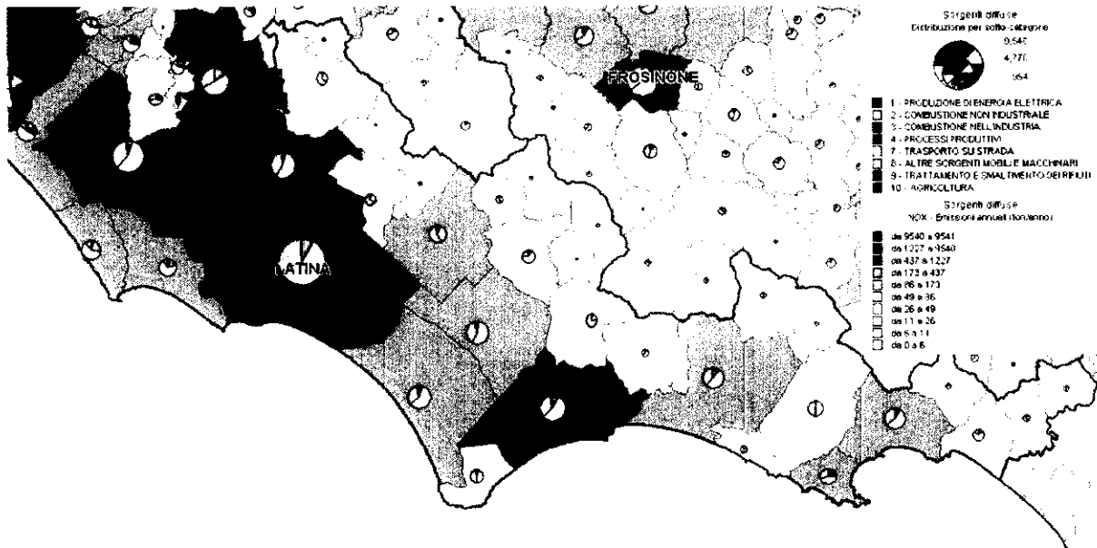
Figura 2.7 - Contributo dei macrosettori alle emissioni di NOx della provincia di Latina.
