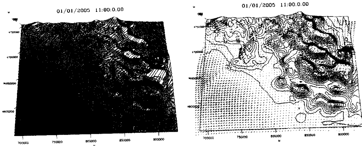
Figura 3.19 - Linee di flusso (sinistra) e campo di vento corrispondente (destra) in prossimità del suo-lo relativi al giorno 1/1/2005 alle ore 11:00 simulati attraverso la catena RAMS/ISAN – GAP sull'area del Lazio.
