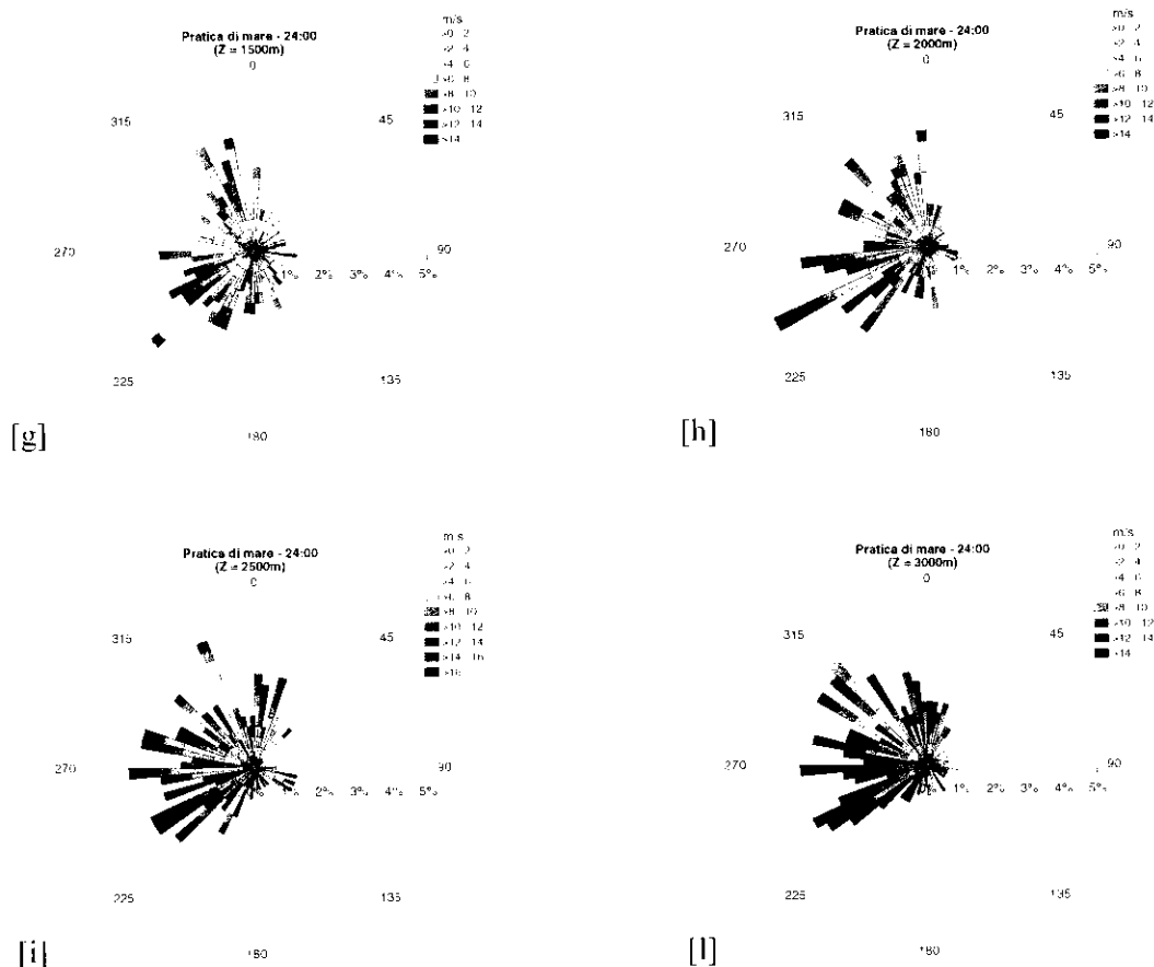
Figura 2.45 - Rilevazioni effettuate con i radiosondaggi a Pratica di mare relative alle 24:00 nel 2005.
