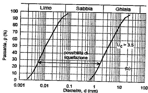
Fig. 1b – Distribuzione granulometrica con terreni con U_c > 3.5
