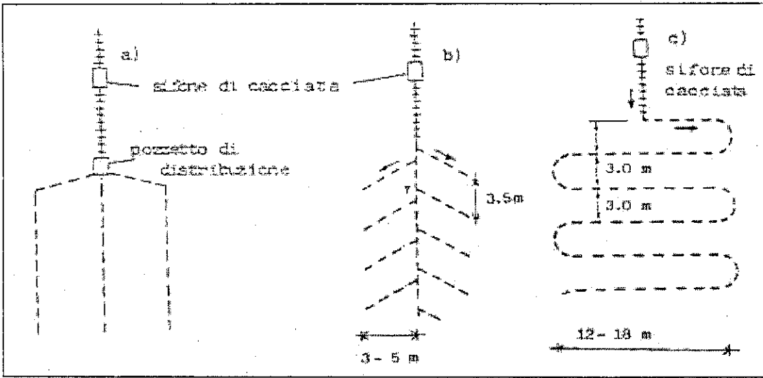
Disposizione delle condotte di sub-irrigazione (Frangipane - Vismara, 1994)
