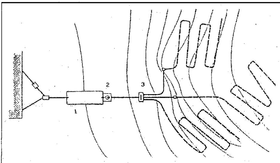
Andamento planimetrico delle condotte di sub-irrigazione (Frangipane - Vismara, 1994)
