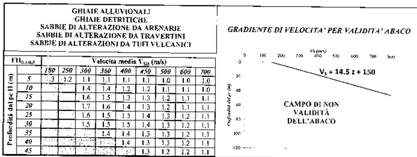
Fig. 1: Abaco per le Ghiaie alluvionali, detritiche e Sabbie di alterazione
