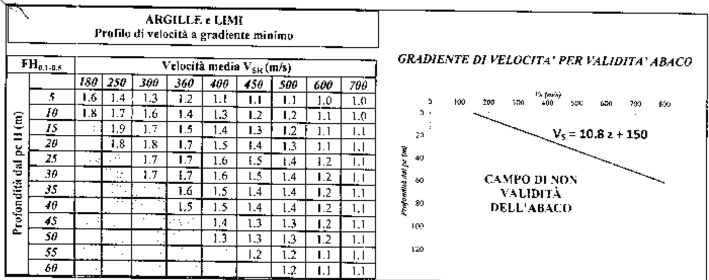
Fig. 4: Abaco per le Argille e Limi con gradiente di velocità minimo
