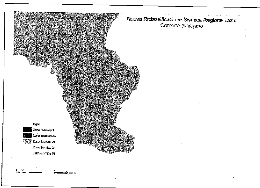
Riclassificazione Sismica per il Comune di Vejano suddiviso in due sottozone sismiche. L'Isola Amministrativa è in sottozona 2B mentre il Comune in sottozona 3A
