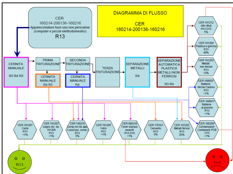
Linea 1 - Trattamento rifiuti non pericolosi da apparecchiature elettriche ed elettroniche
