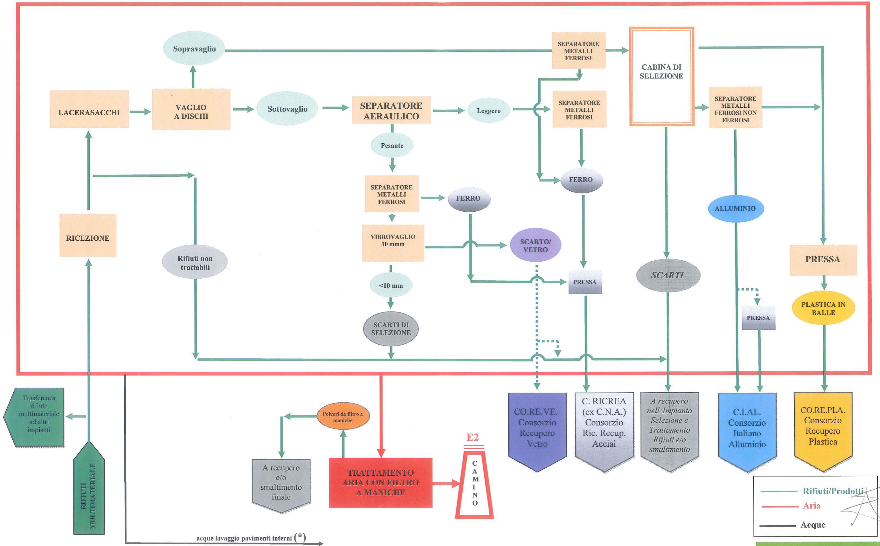
Figura 1. Schema a blocchi del processo Assetto Futuro
