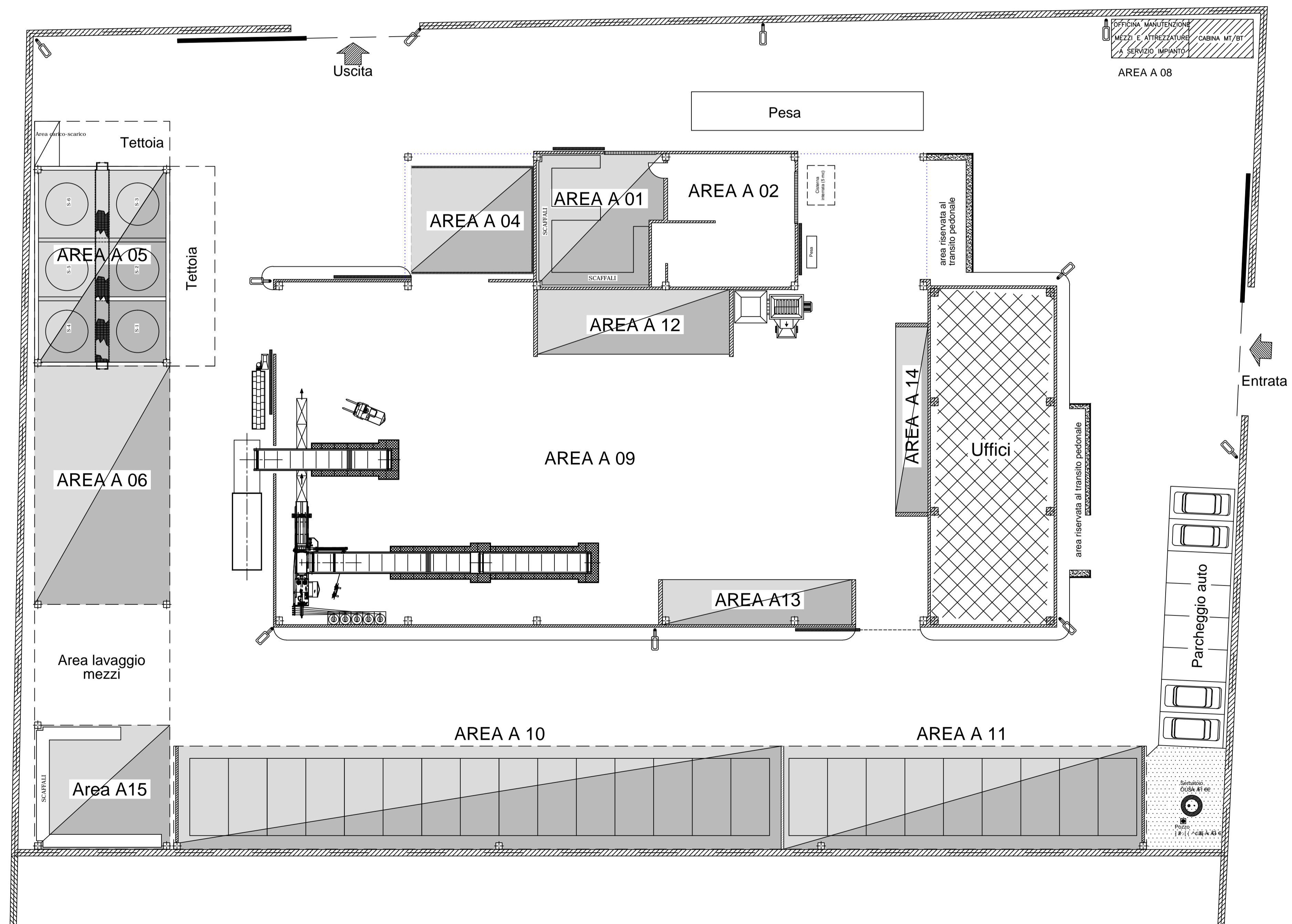
PLANIMETRIA GENERALE 1:200
