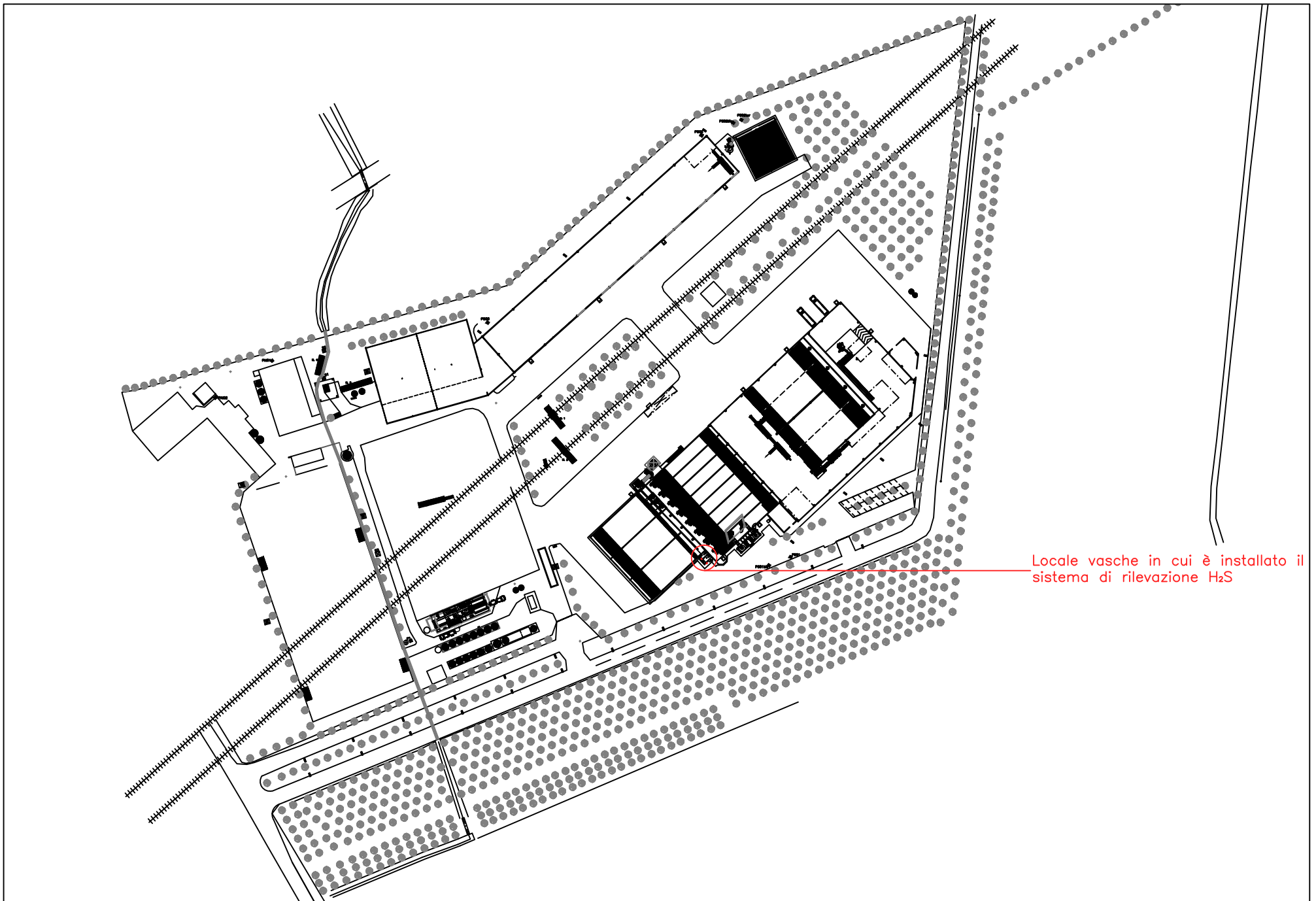
Key-plan impianto KYKLOS con evidenziato il locale vasche in cui è stato installato il sistema di rilevazione H 2 S
