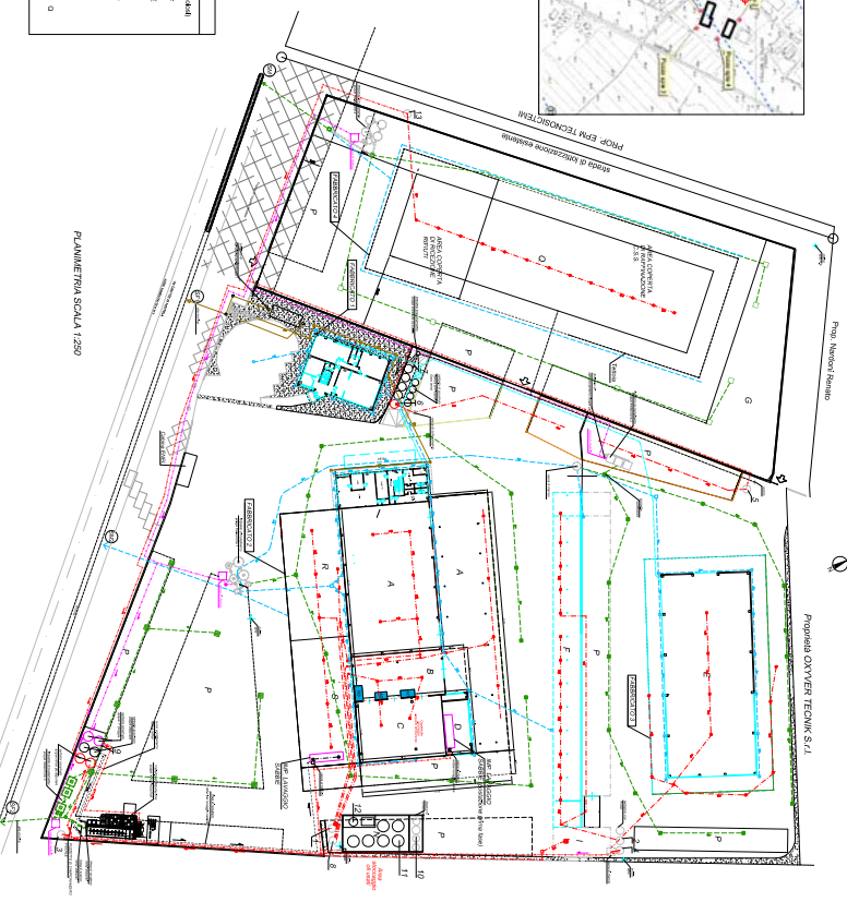
IMPIANTO DI DEPURAZIONE BIOLOGICA FANGHI ATTIVI
