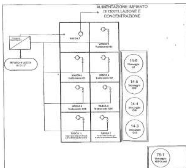
Schema di processo richiesto per l'utilizzo delle vasche e dei serbatoi di stoccaggio e trattamento
