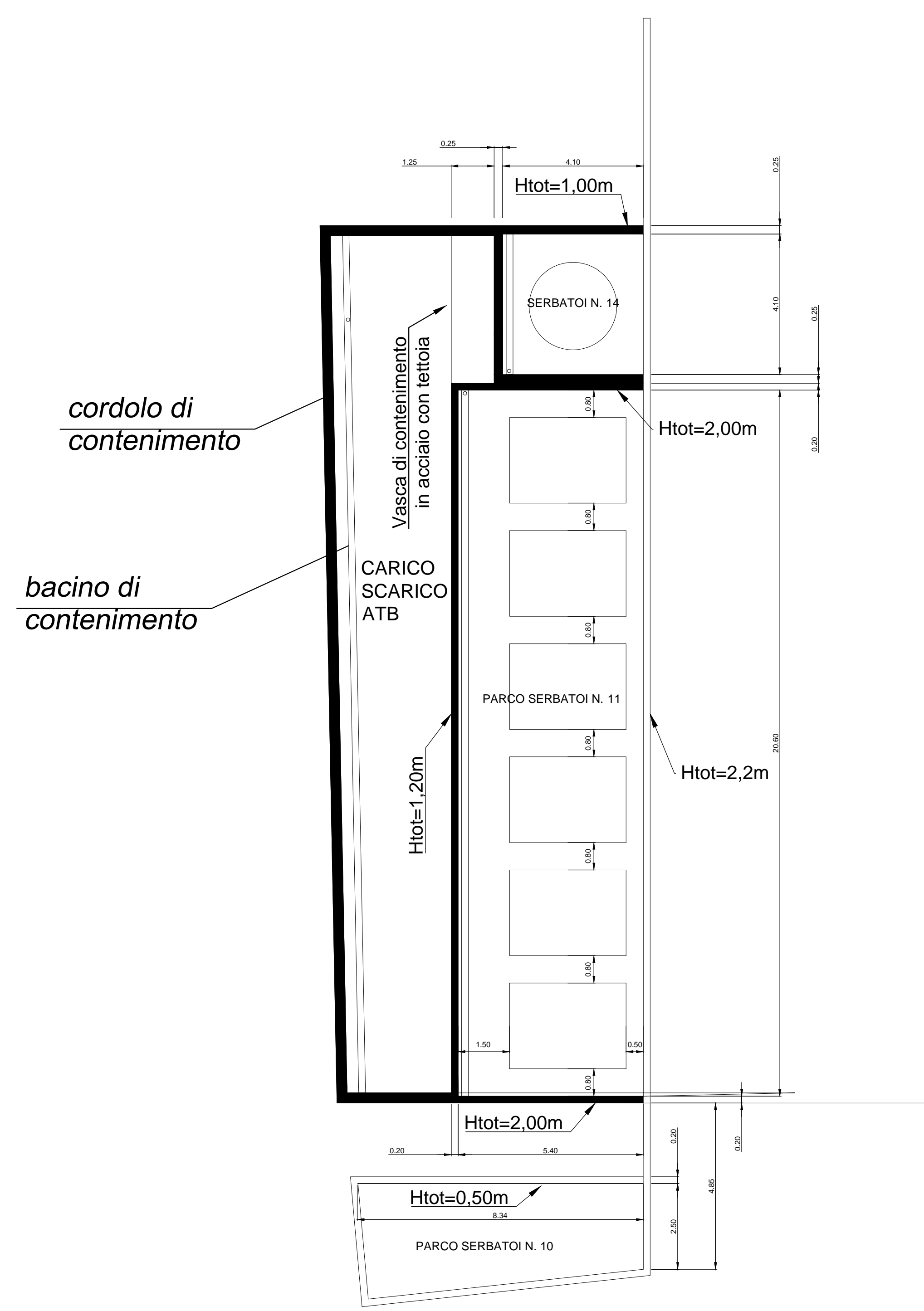
PIANTA SCALA 1:100
